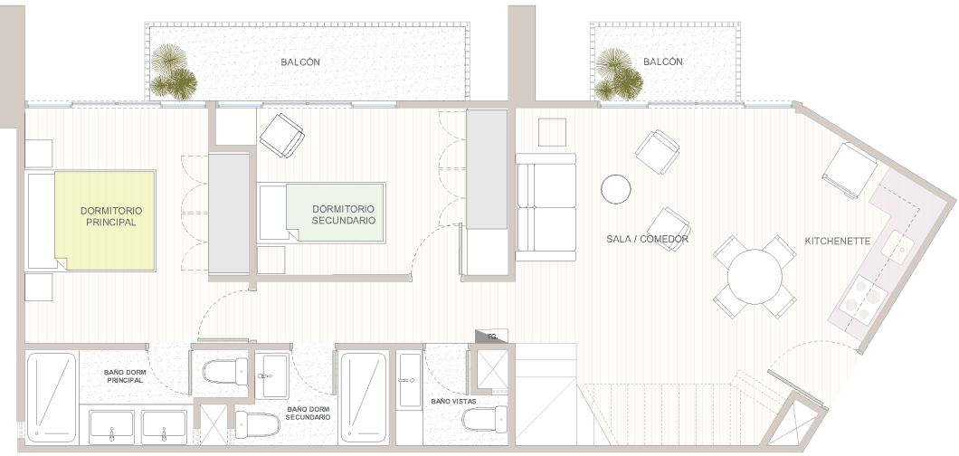
PRIMER NIVEL
